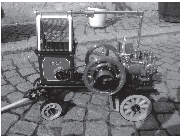
Kutil pan Jiří Blaha (43) z Věže si splnil životní sen a doma sestavil plně funkční model stabilního motoru. Práce na stroji trvala čtyři roky, ale výsledek stojí za to. Shlédnout video můžete na www.youtube.com , poté hledat - motor stabilák Jiří Blaha.
